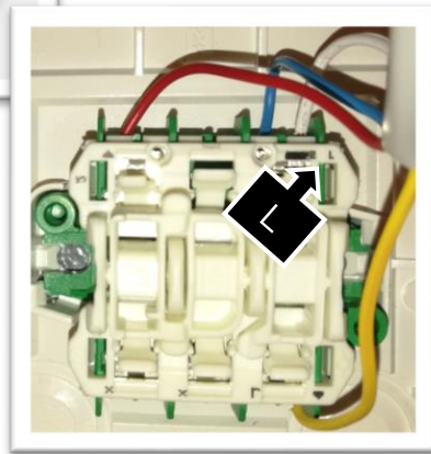
Kuva 1. KLM 4x0.8:n johtimien kytkentä VMSW-S -kytkimellä.
